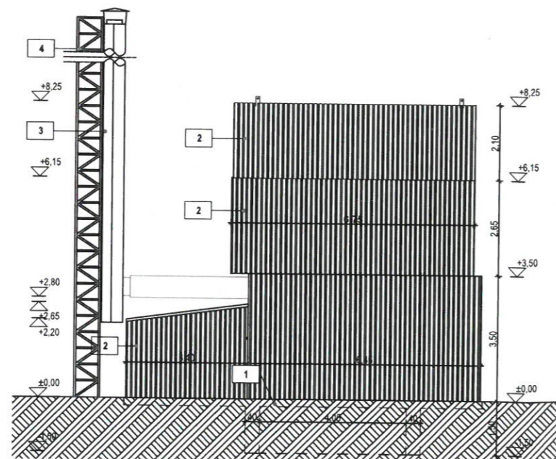
NYUGATI HOMLOKZAT M 1:100
