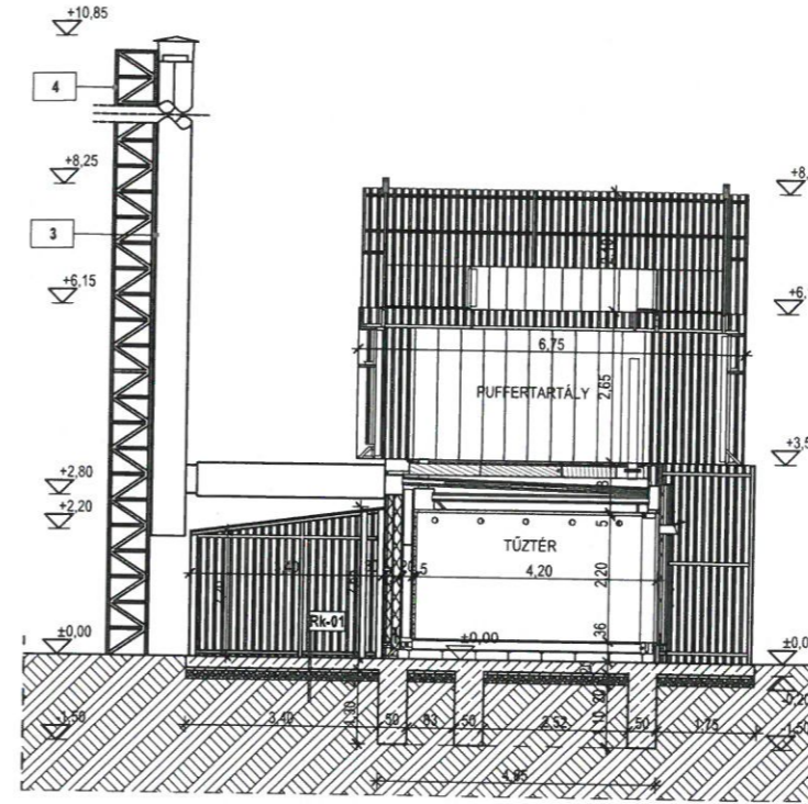
METSZETEK M 1:100
