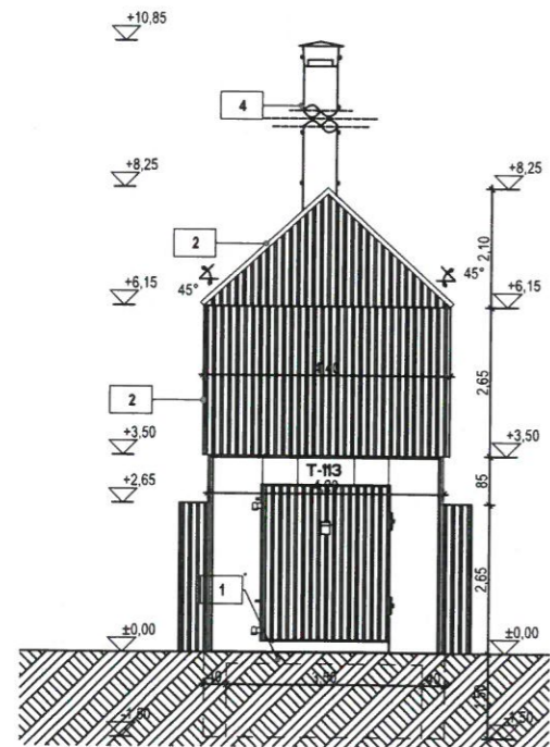
DÉLI HOMLOKZAT M 1:100
