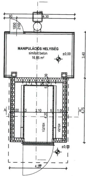
ALAPRAJZ, M 1:100 +1,00 m METSZŐSÍKON
