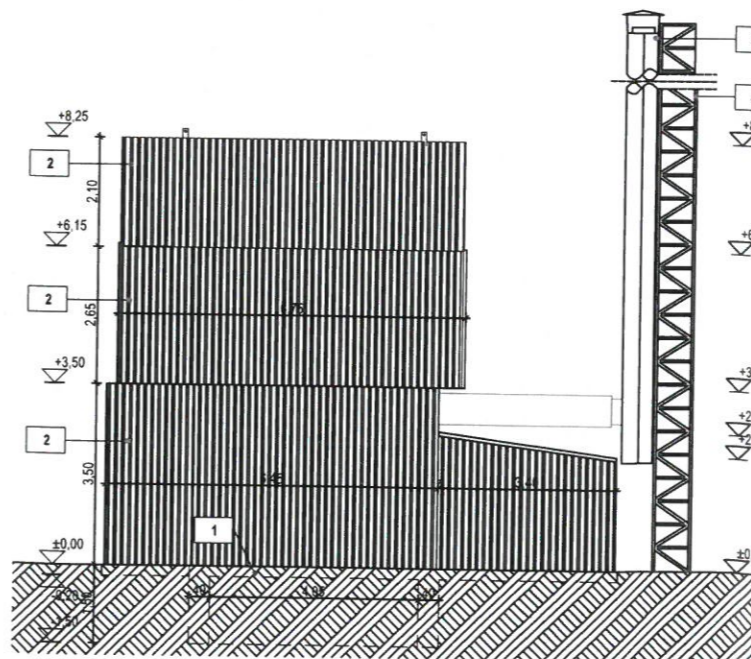
KELETI HOMLOKZAT M 1:100
