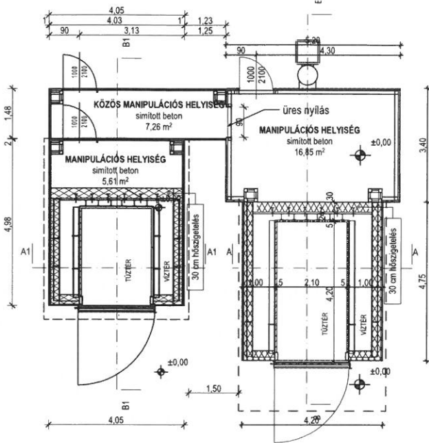
ALAPRAJZ, M 1:100 +1,00 m METSZŐSÍKON
