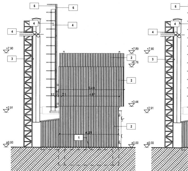
NYUGATI HOMLOKZAT M 1:100
