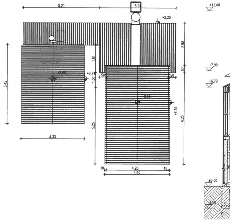
FELÜLNÉZET M 1:100
