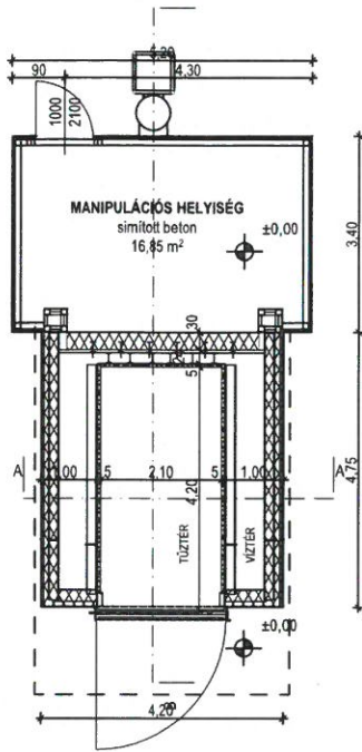
ALAPRAJZ, M 1:100 +1,00 m METSZŐSÍKON
