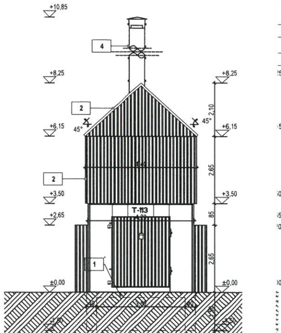
DÉLI HOMLOKZAT M 1:100
